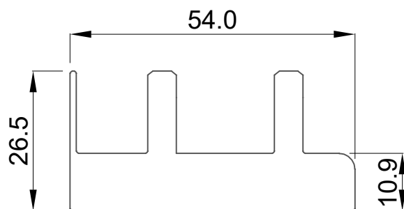
FI-3880 MARCO 2 RIELES
