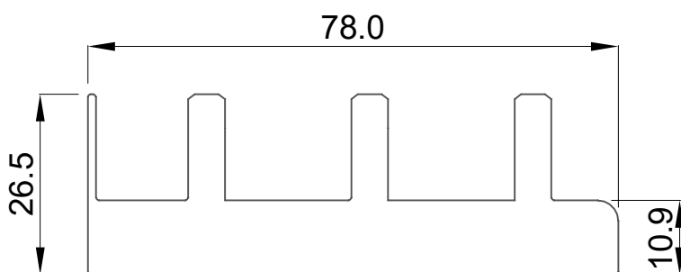
FI-4632 MARCO 3 RIELES
