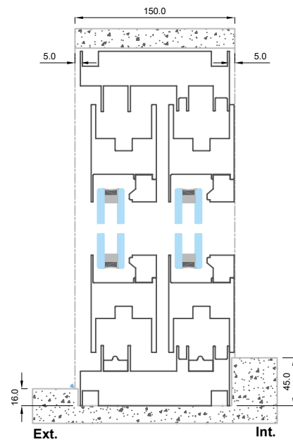
Sección B-B'
