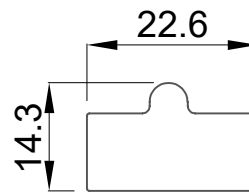
FI-5932 RIEL
