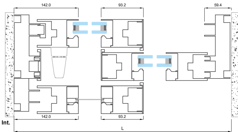
Sección A-A' Ext.
