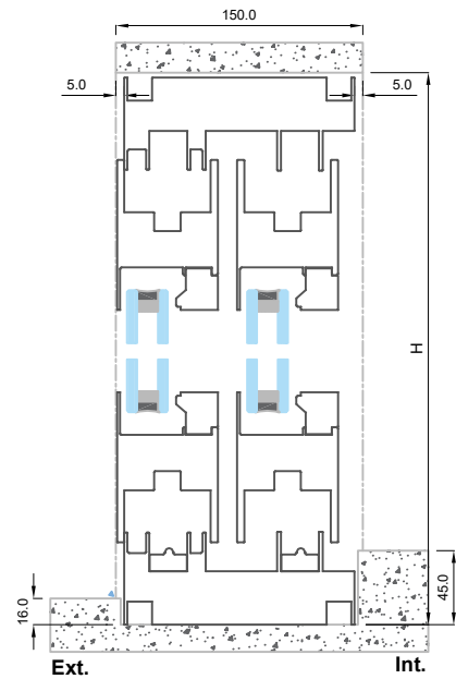
Sección B-B'
