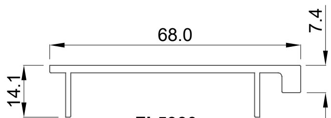
FI-5930 TAPA DE HOJA
