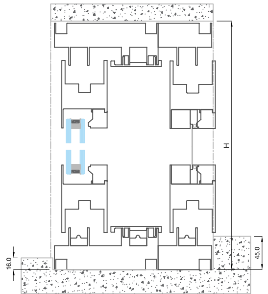
Sección B-B'
