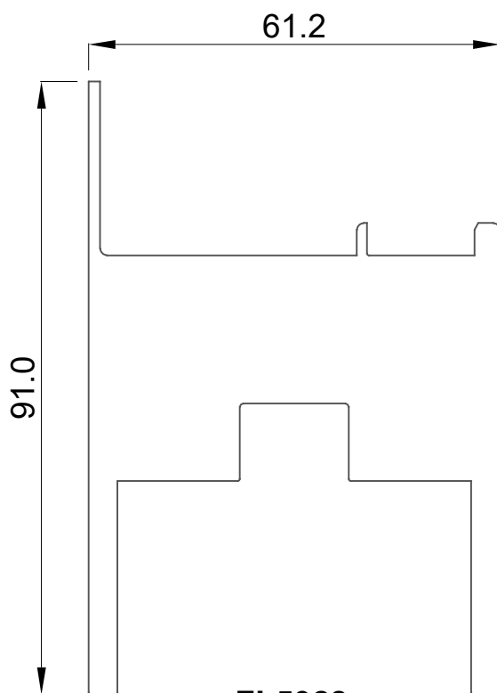
FI-5928 HOJA
