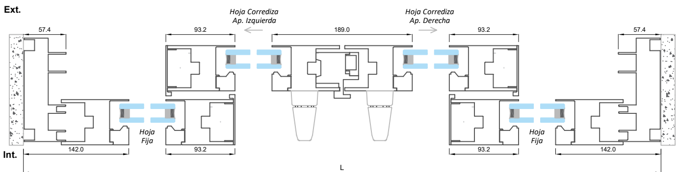
Sección A-A'
