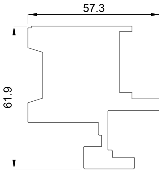
FI-5949 ADAPTADOR DE HOJAS
