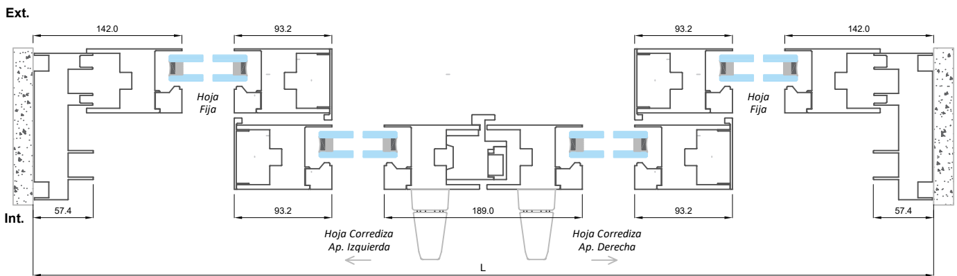
Sección A-A'
